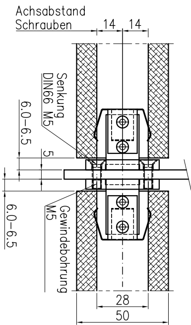
Montage beidseitig am Fassadenprofil
